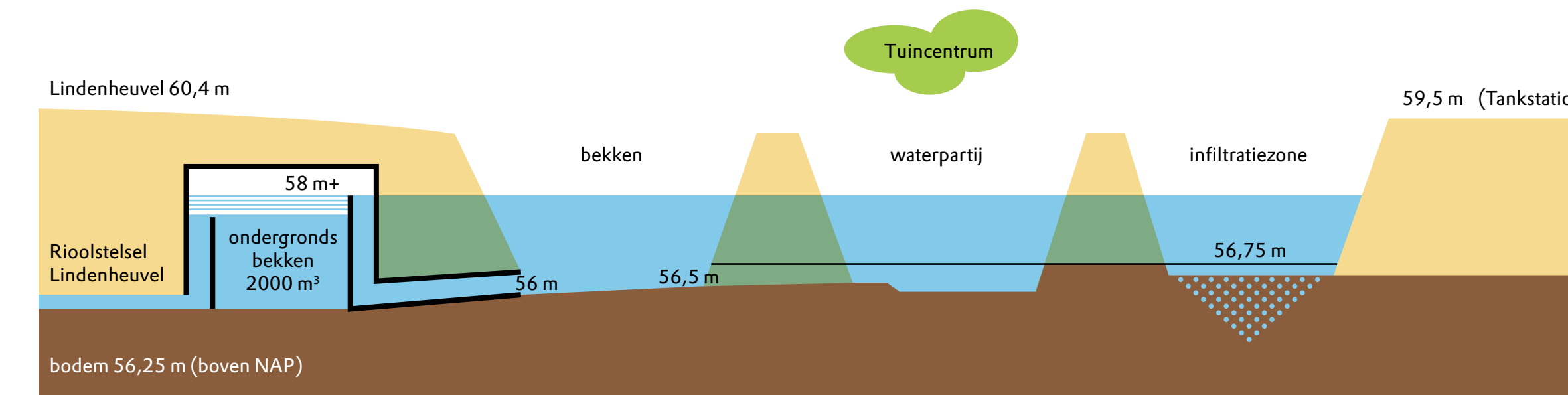
Watersysteem 'Hof van Limburg' in relatie tot het rioolsysteem Lindeneuvel.
